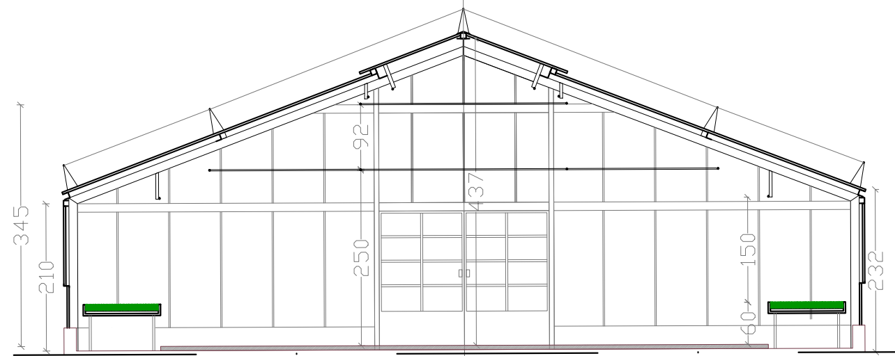
Sez A-A
