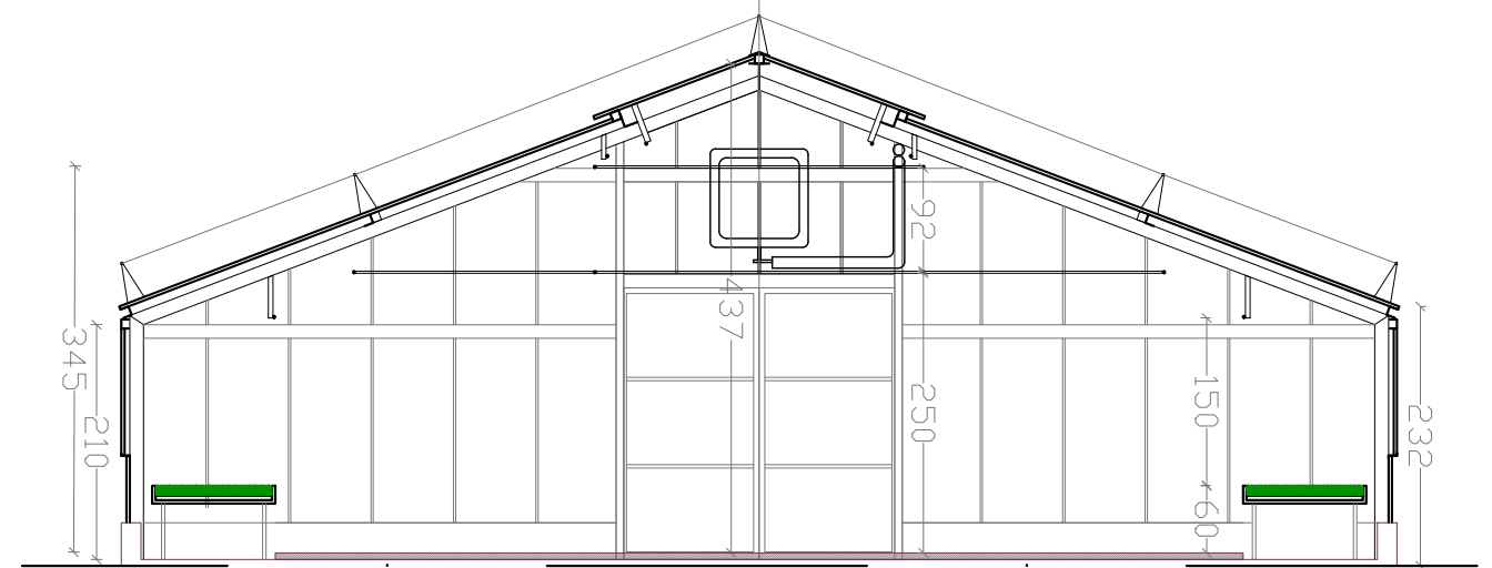
Sez B-B
